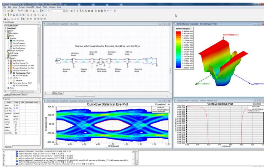
SPパラメータを含む回路でトランジェント解析を行いアイパターンを表示
