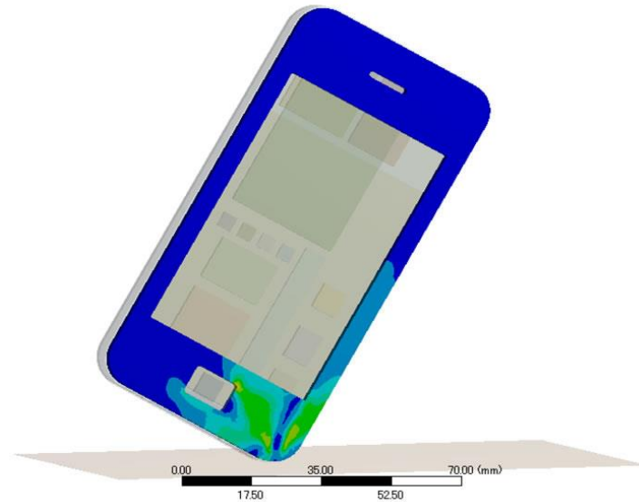
スマートフォンの落下（陽解法過渡解析）
