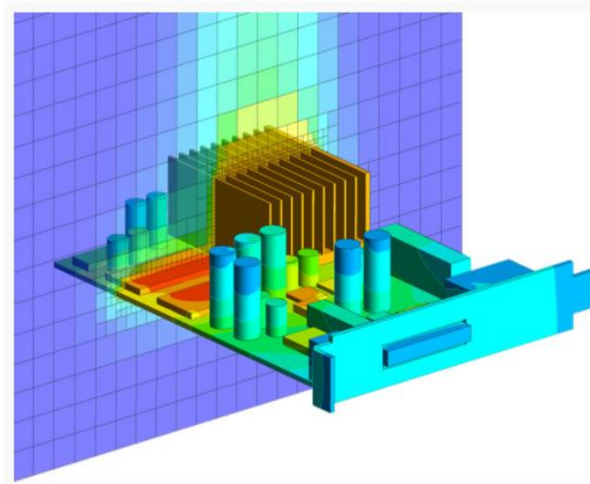
グラフィックボードの熱流体解析
